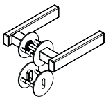
CUBICO PIATTA R Schlüsselrosetten BB CUBICO PIATTA R Roses BB
