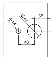
Bohrungen Schlosskasten Bores glass-door lock
