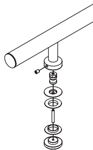
Adapterset zur einseitigen Montage Holztüren (mit Gegenplatte) Adapter set for unilateral installation, wood doors (with strike plate)
