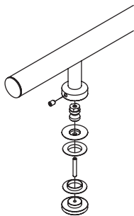
Adapterset zur einseitigen Montage Glastüren (mit Gegenplatte) Adapter set for unilateral installation, glass doors (with strike plate)
