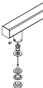
Adapterset zur einseitigen Montage Glastüren (mit Gegenplatte) Adapter set for unilateral installation, glass doors (with strike plate)
