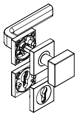
GRAPH Schraub Wechselgarnitur eckig Ausführungen: PZ, RZ mit Knopf Square GRAPH screw rose change square set Options: PZ, RZ with knob square
