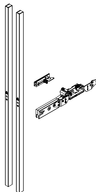
PLANEО GS_49017 smart2lock Ausführung: Rechts öffnend PLANEО GS_49017 smart2lock option: right opening
